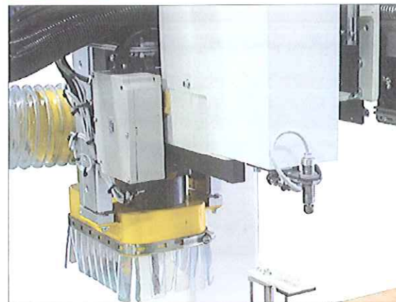
マガジンプッド（最大5個） 工具長センサー（オプション）
