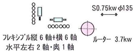
TW-267P-II RS 軸構成
